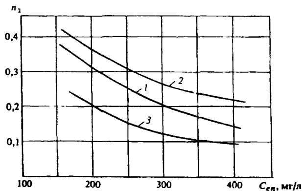
Черт. 2. Зависимость показателя степени n_2 от исходной концентрации взвешенных веществ в городских сточных водах при эффекте отставания
