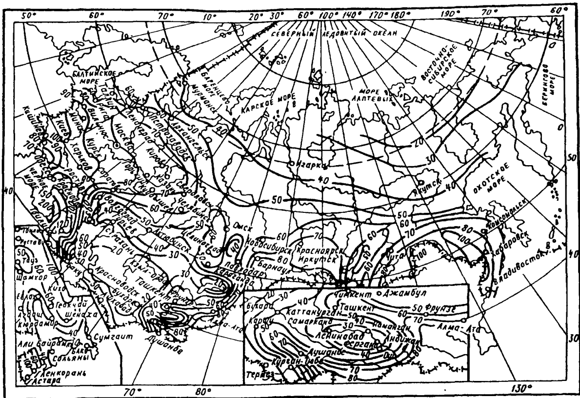
Черт. 1. Значения величин интенсивности дождя q_{20}
